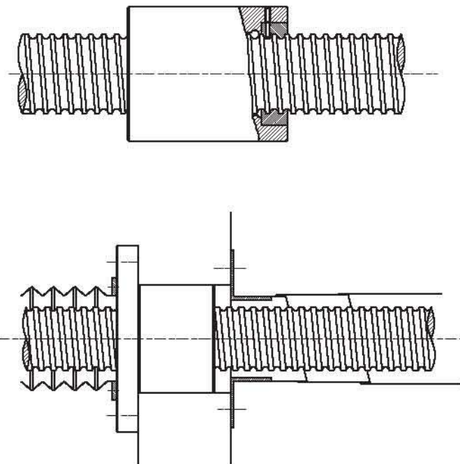
圖 5.1 防塵機構
