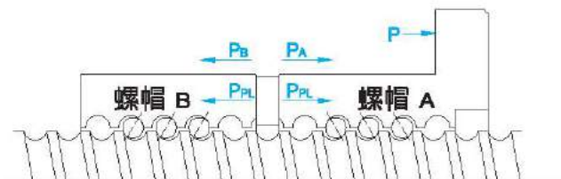
■ 3.29 雙螺帽預壓負荷
