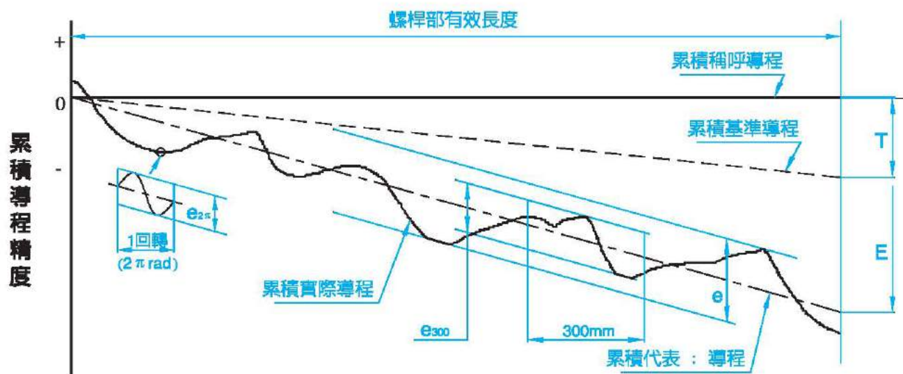
■ 3.1 導程精度之說明圖
