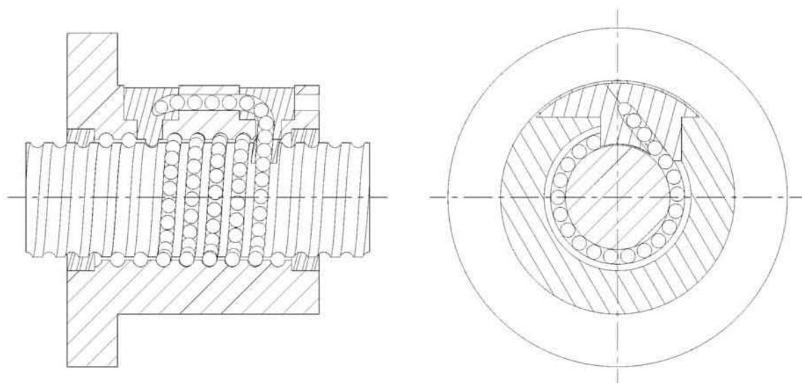
■ 3.24 V 型螺帽 ■
