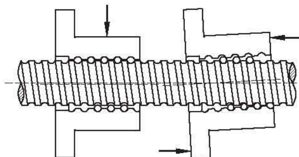
圖 5.2 偏荷重
