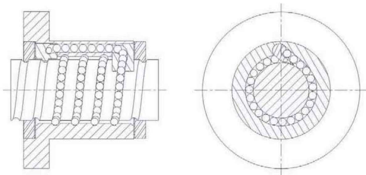
■ 3.23 S 型螺帽 ■
