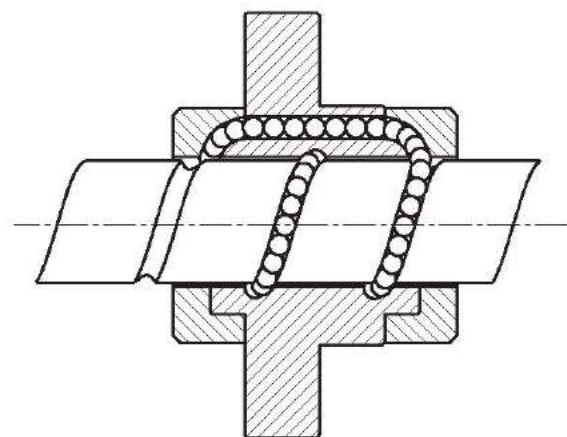
■ 3.28 E 型螺帽圖
