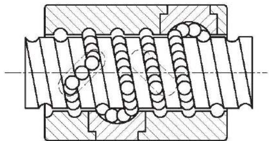
■ 3.26 U.I 型螺帽圖
