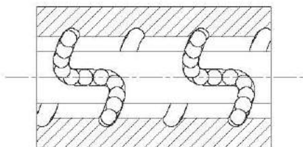
■ 3.27 K 型螺帽圖
